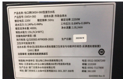
铭牌
