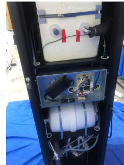
内部结构
