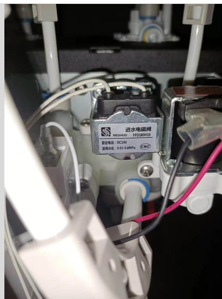
进水电磁阀
